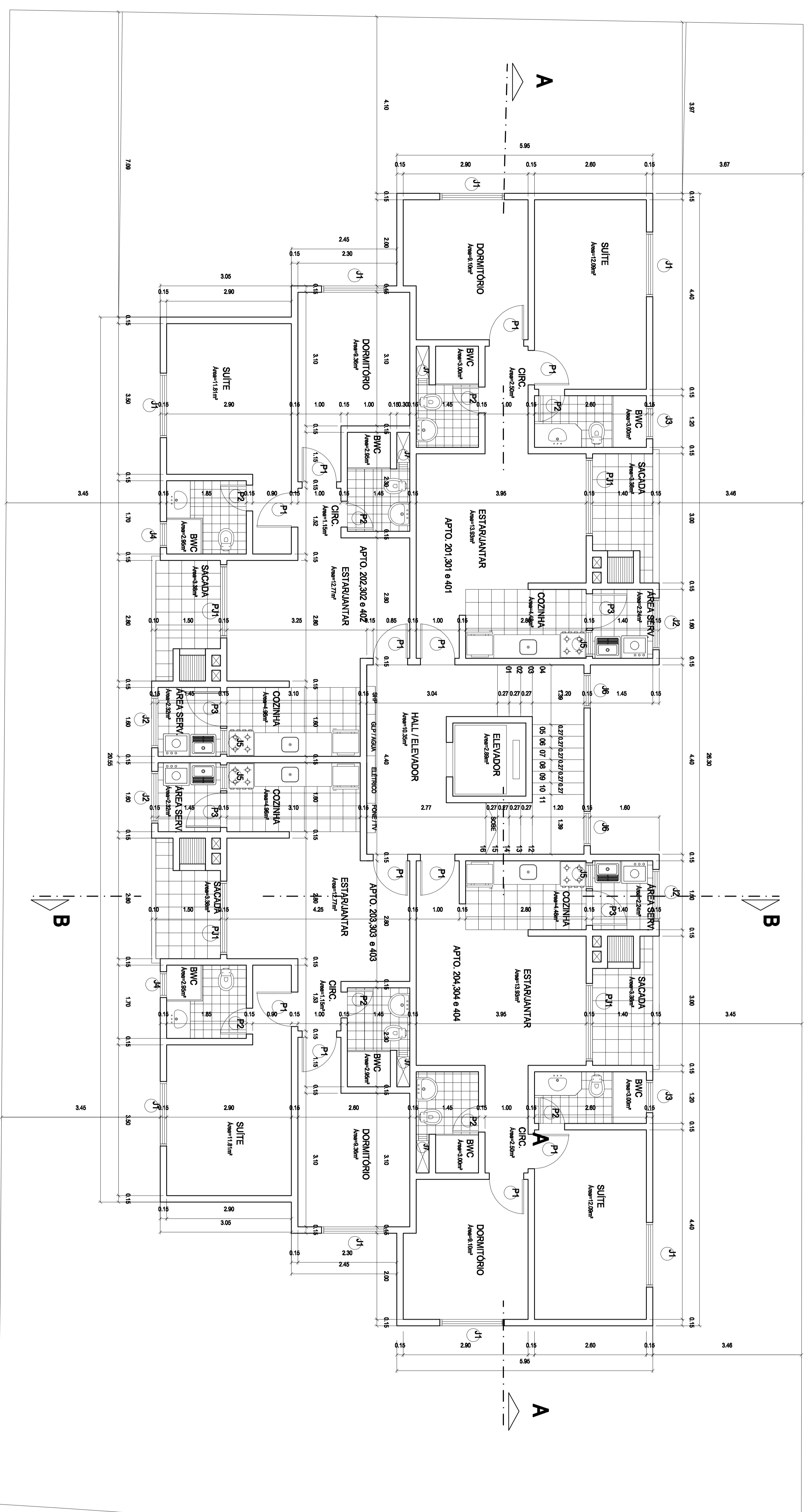
PLANTA BAIXA - PAVTO. TIPO (X3)
